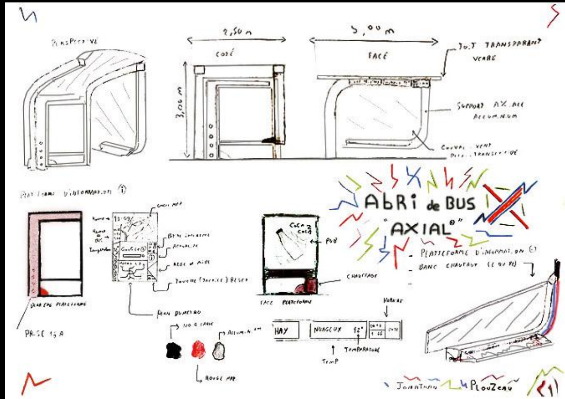
Jonathan PLOUZEAU - 1BPE - Abris de bus actuel "Axial"
