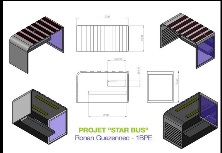
Ronan GUEZENNEC - 1BPE - Abris de bus futuriste "StarBus" - Du croquis à l'expression en 3D
