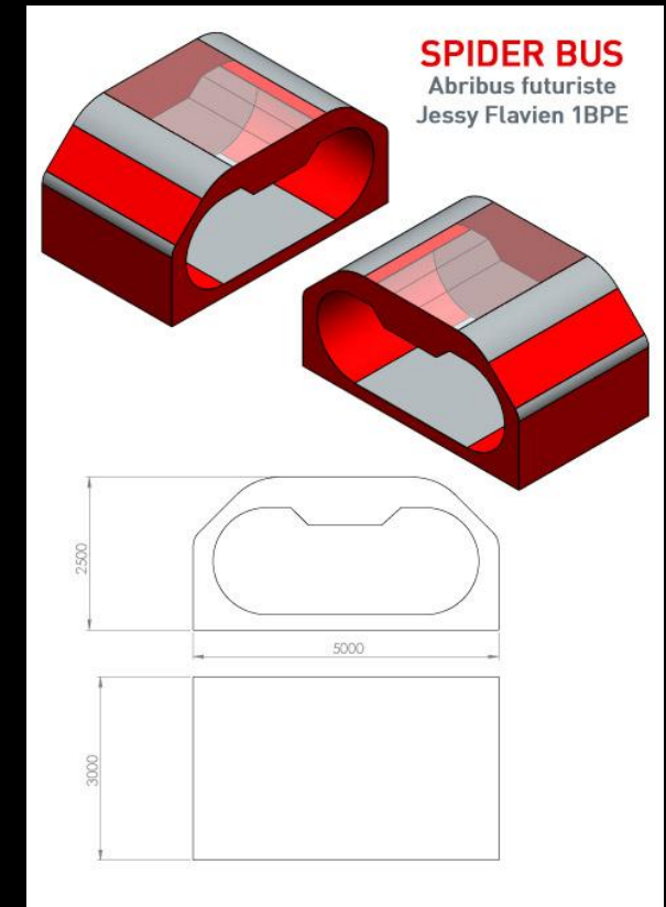
Jessy FLAVIEN - 1BPE - Abri de bus futuriste "Spider-Bus" - Du croquis à l'expression en 3D
